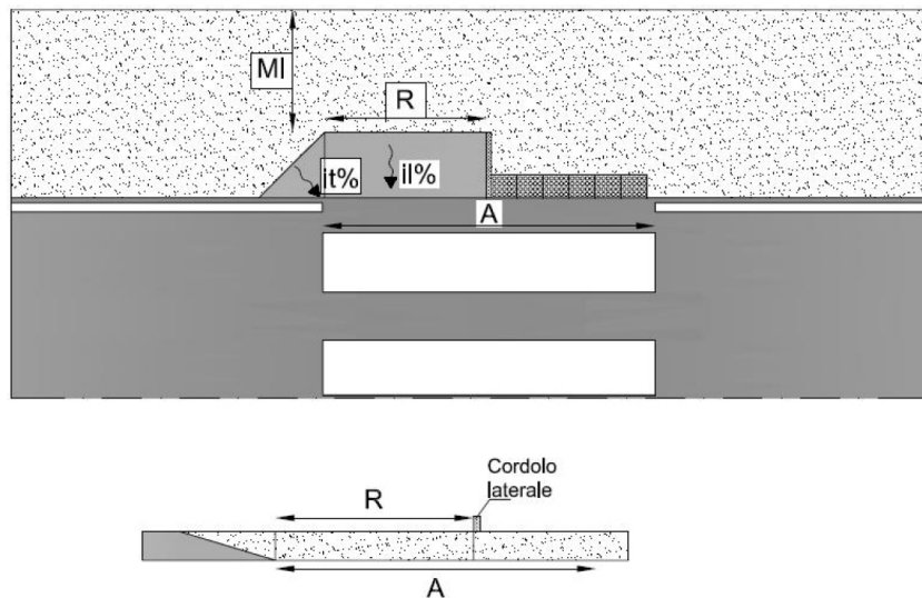
SCHEMA 2a – RAMPA PERPENDICOLARE AL SENSO DI MARCIA DEI VEICOLI
