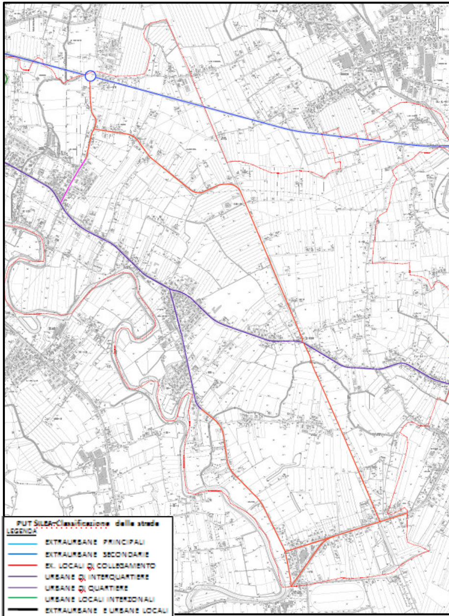
Fig. 3.1.b – Classificazione delle strade principali: CENDON E SANT'ELENA
